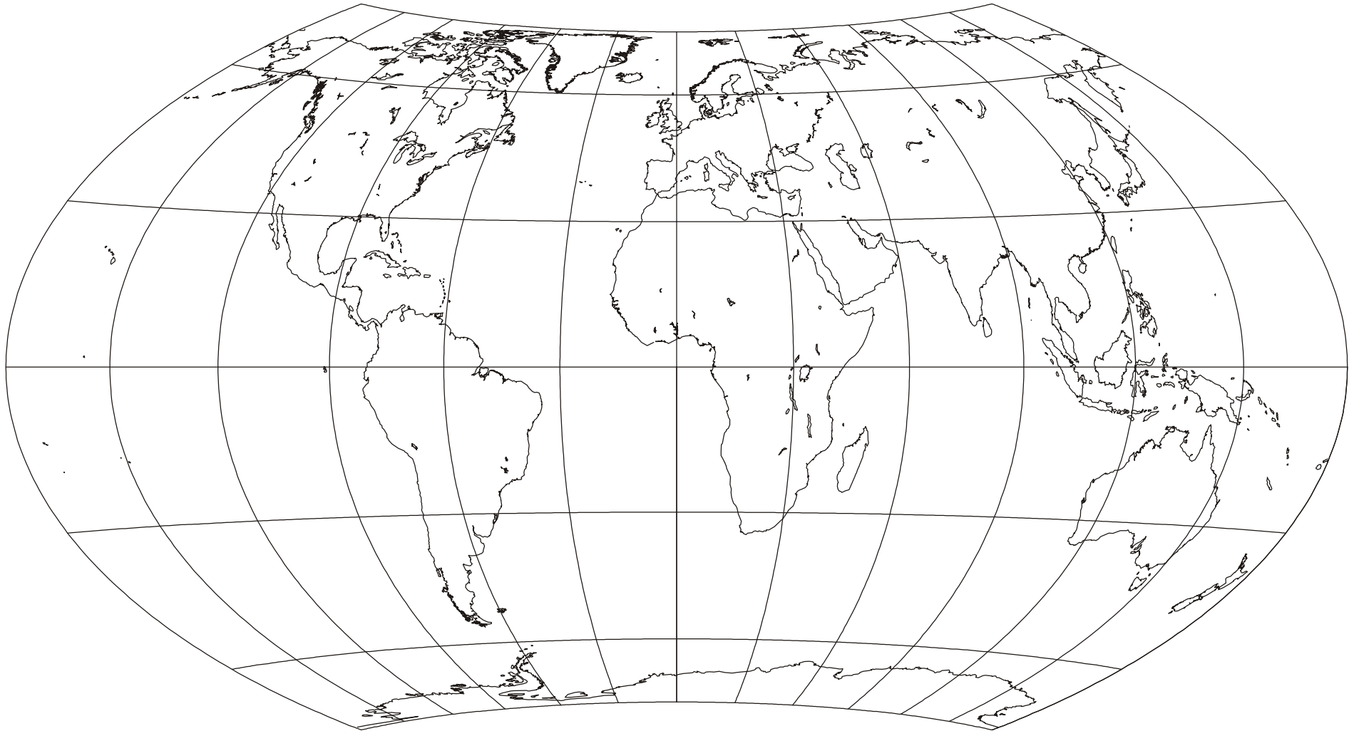
Wagner VII (Hammer-Wagner); Azimuthal; Equal-area; K. H. Wagner, 1941
